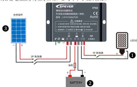
图 2 连接图
