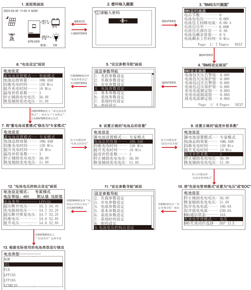
● 图2 “有BMS有充放电末端电流控制设置流程”
